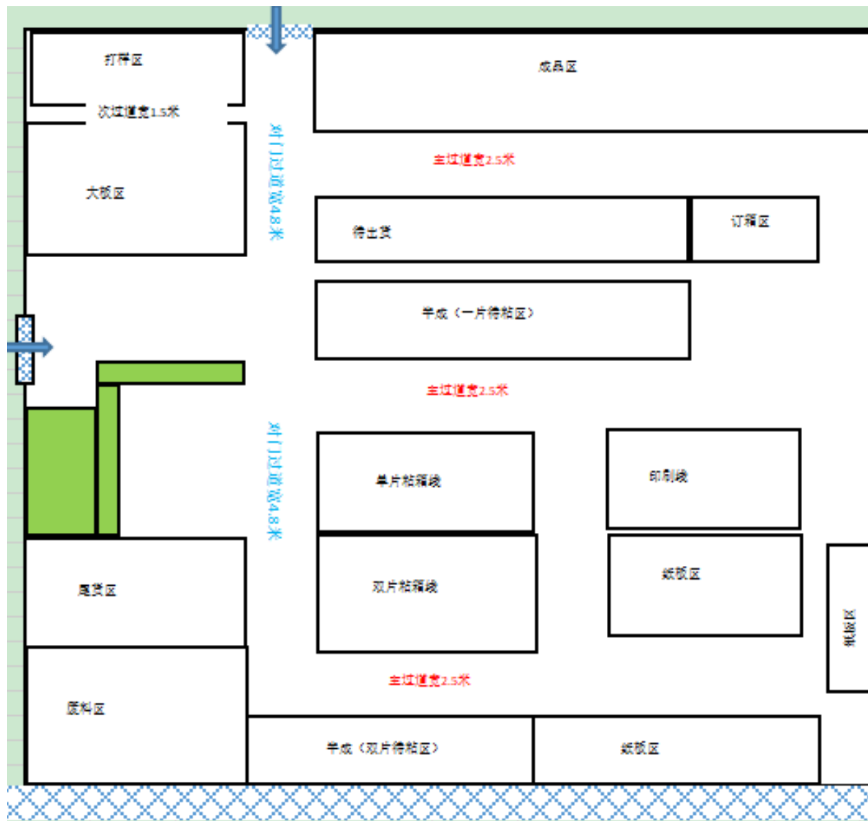
附图3 项目总平面布置图
